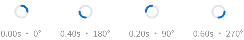
转圈关键帧 · 0.8s linear 无限循环，一周期转 360°（下列 4 帧为 1/4 等分）
